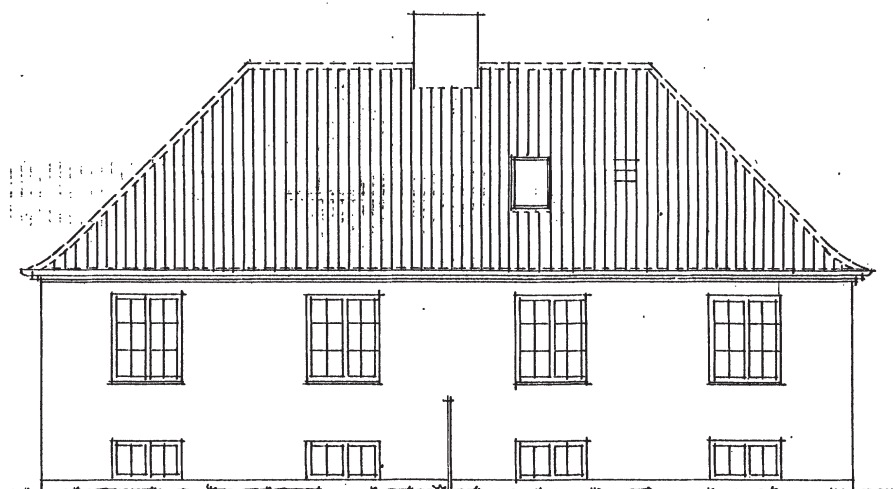
Oprindelig tegning af østvendt facade på bevaringsværdigt hus på Hendriksholms Boulevard.
