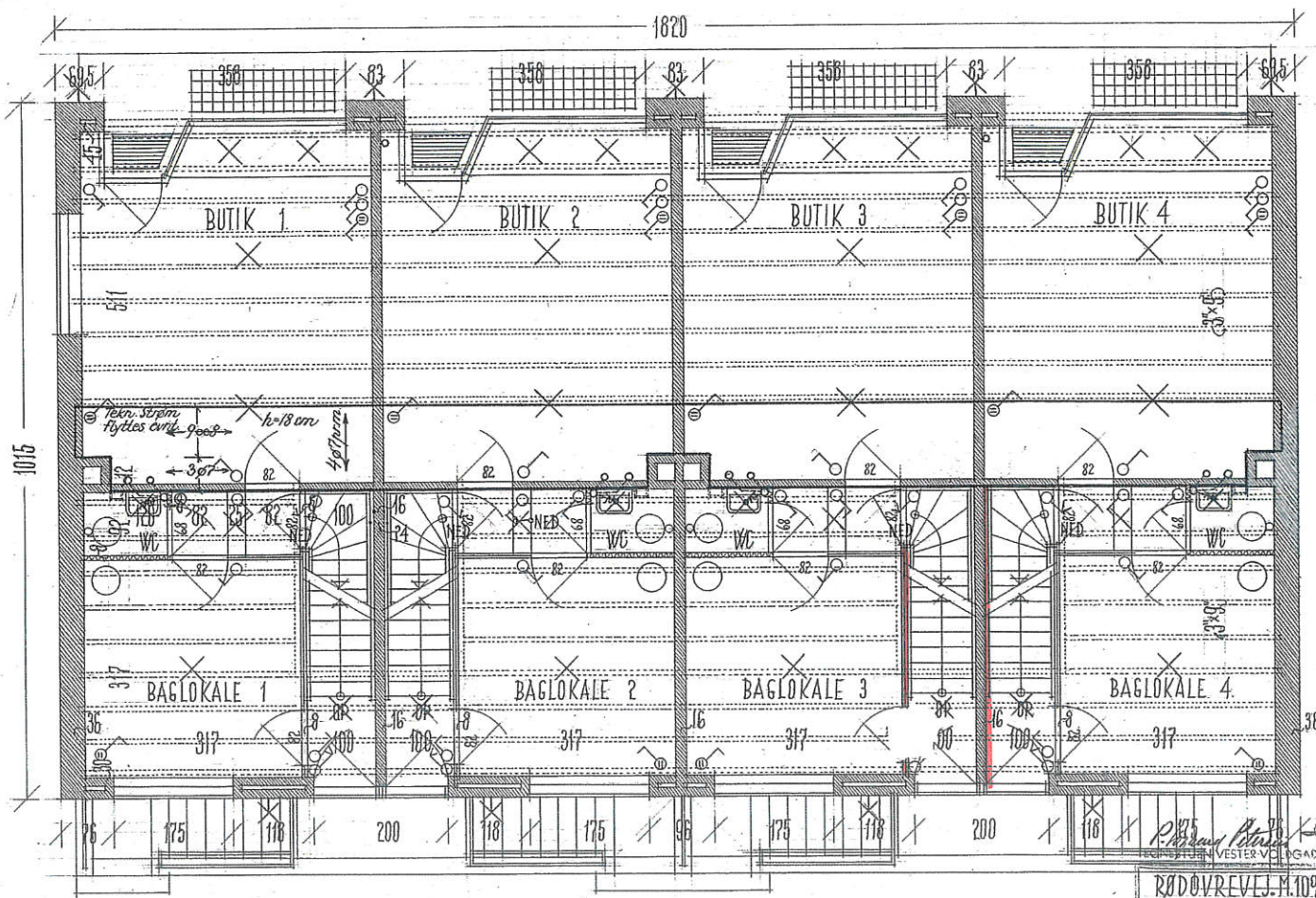
STUEPLAN
