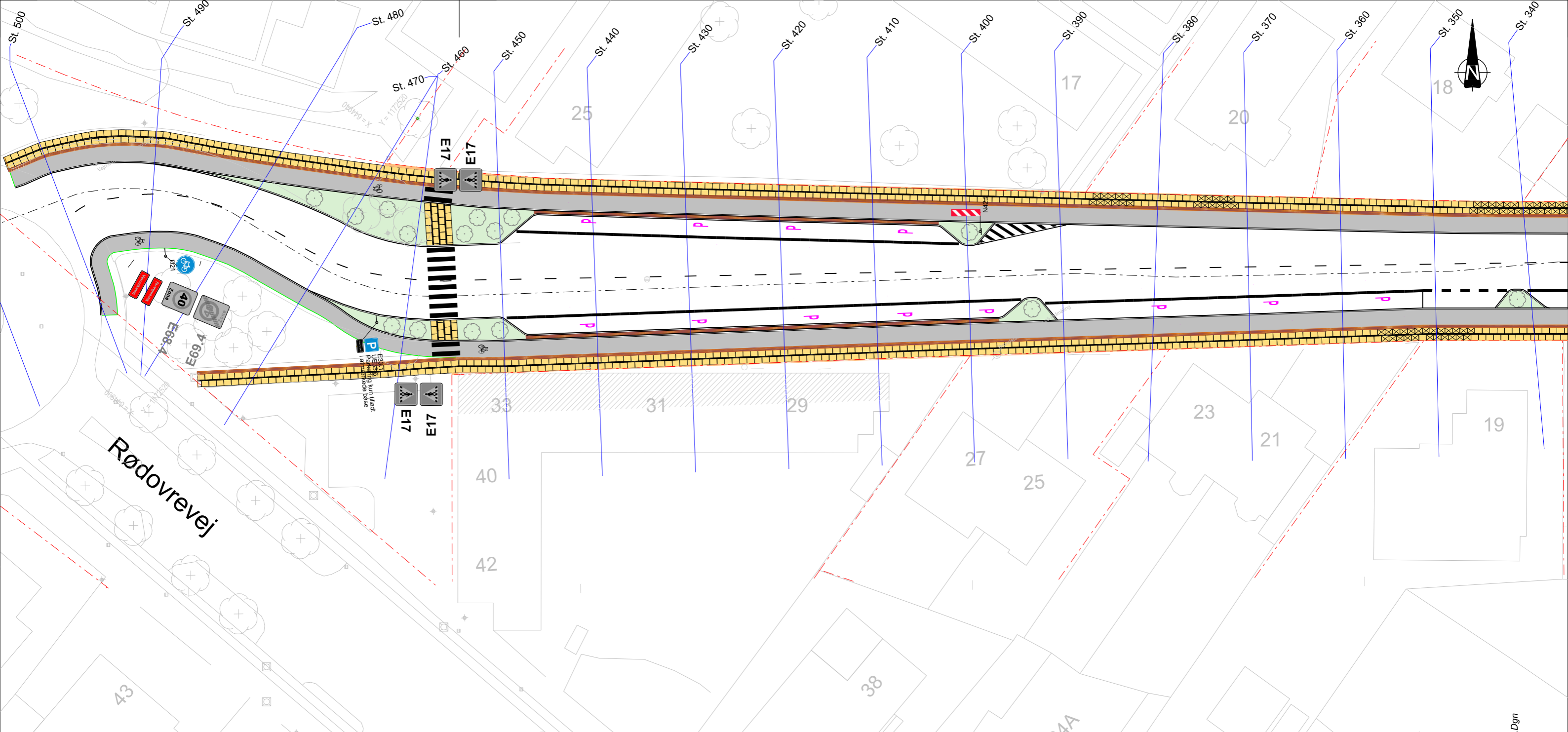
Planudsnit 3 - St. 500 - 340, Størrelsesforhold 1:400
