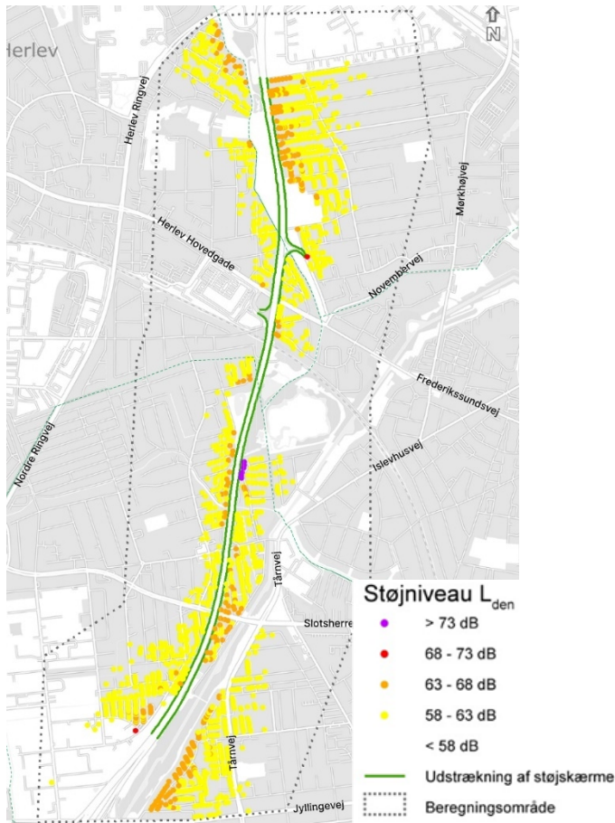
Figur 15 Facadestøj boliger med 8 m støjskærme
