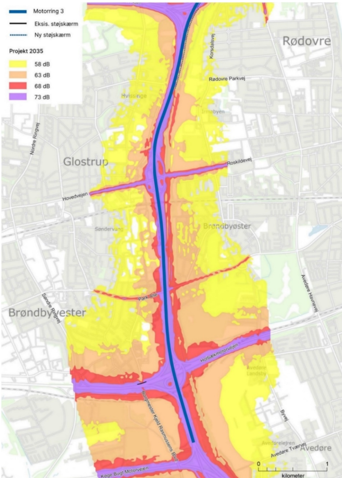
Figur 7 Støjudbredelsen langs Motorring 3 i år 2035, hastighed 90 km/t
